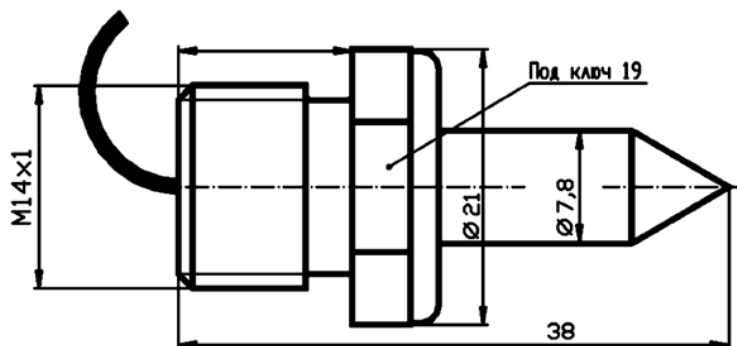
Габаритный чертёж датчика СС06-1
